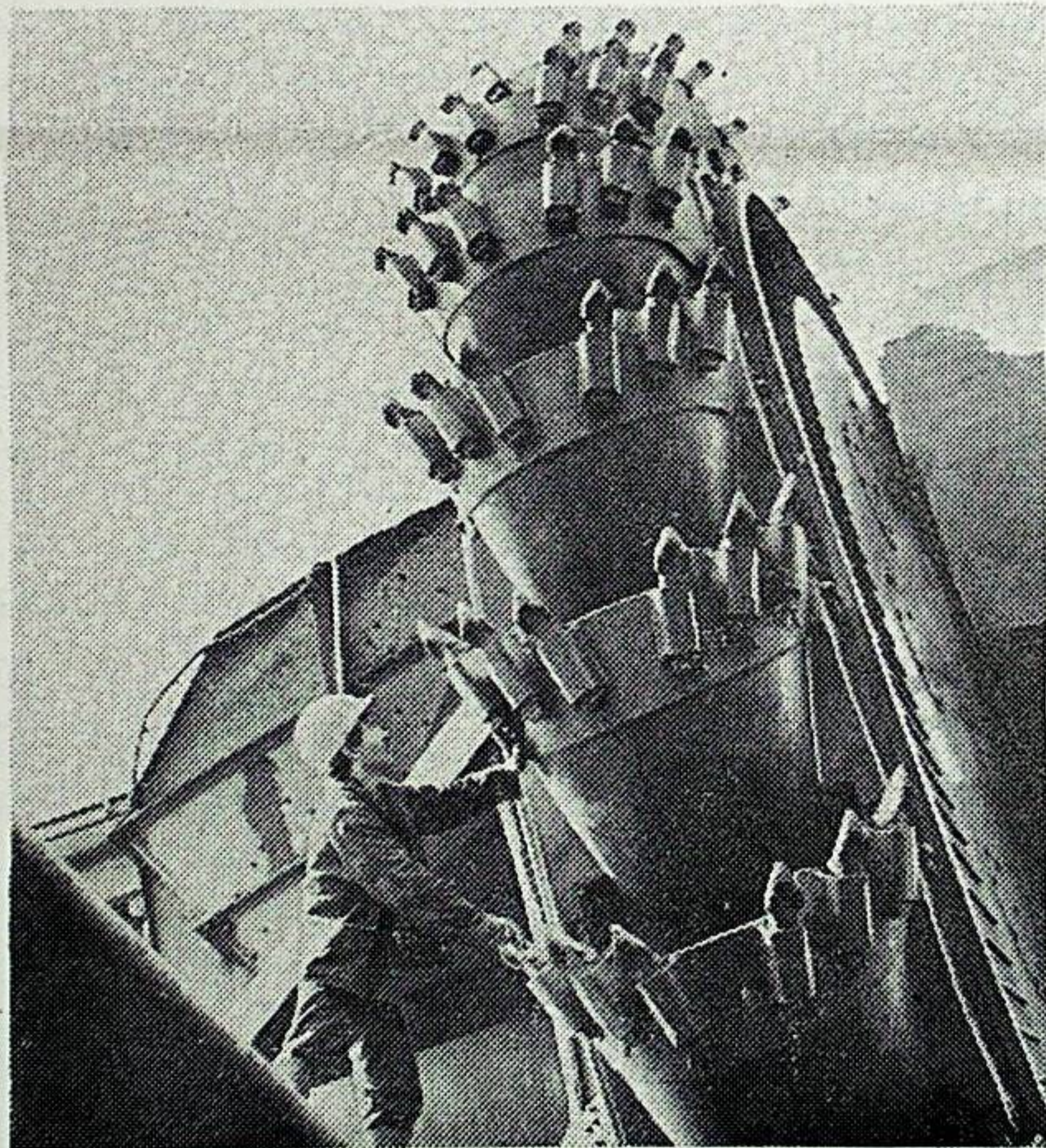
سۈرەتتە: ئېكېباستۇز كۆمۈر يەرلەشمىسىنىڭ «شەمس» شاخىسىدا ئىشلىگۈچى ياردەمچى ماشىنىسىنى باقمىچان زاكىپوۋ ئېكسكاۋاتورنىڭ ئىش ئالدىدىكى ئەھۋالىنى كۆزدىن كەچۈرمەكتە.
