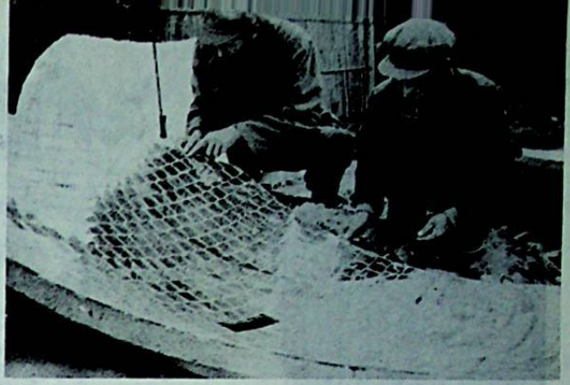
تركيب لوحات المرايا في وجه الفرن الشمسي
