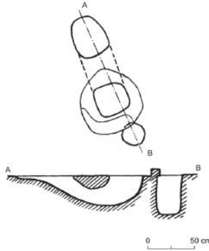
(Resim-53. Ivolga yerleşiminde bulunan fırın yapısının çizimi) 446
